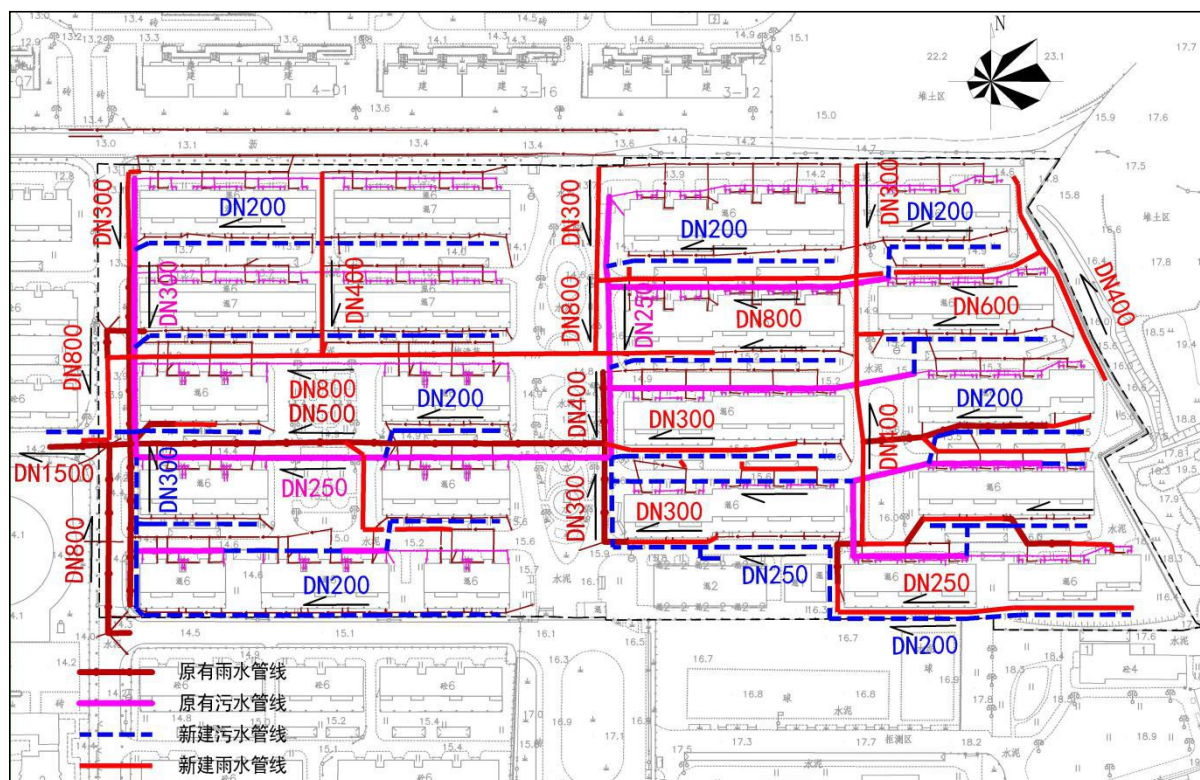
图 2-3 梅清苑排水方案示意图
