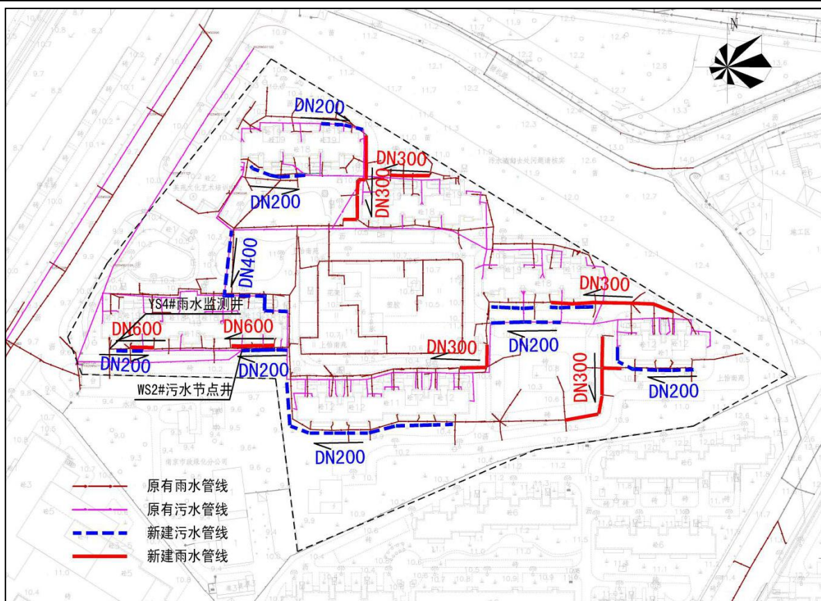
图 2-11 上怡南苑排水方案示意图
