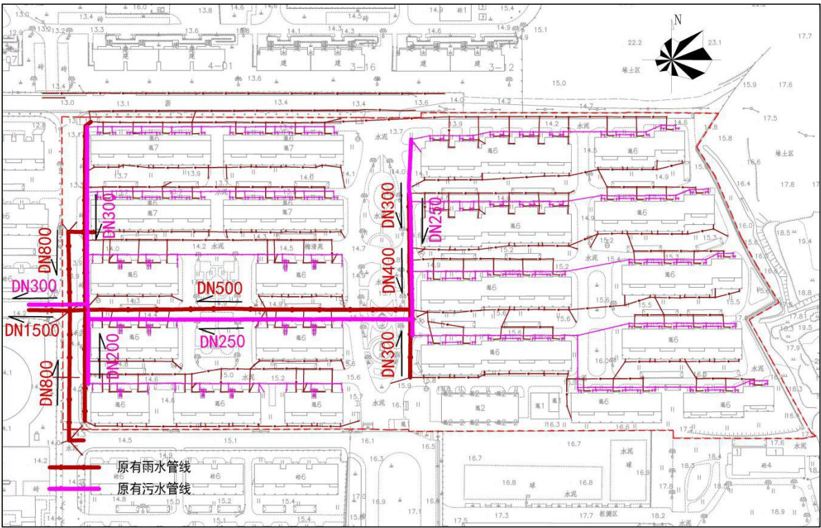
图 2-2 梅清苑排水现状示意图
