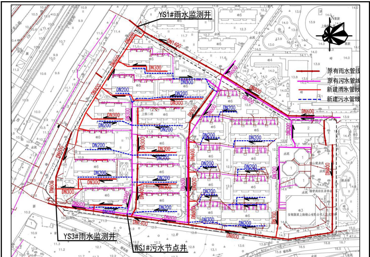
图 2-7 梅秀苑排水方案示意图
