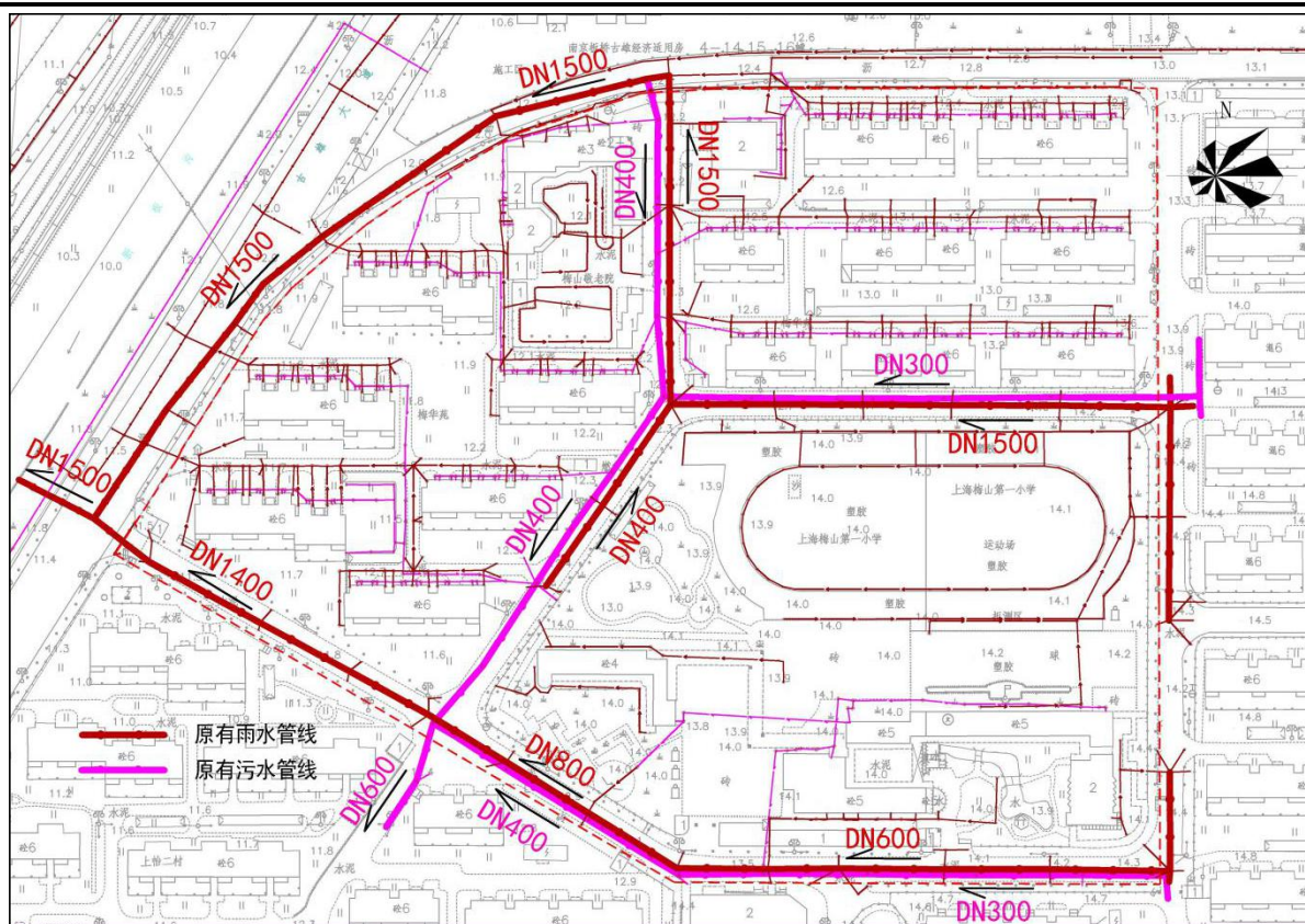
图 2-4 梅华苑排水现状示意图
