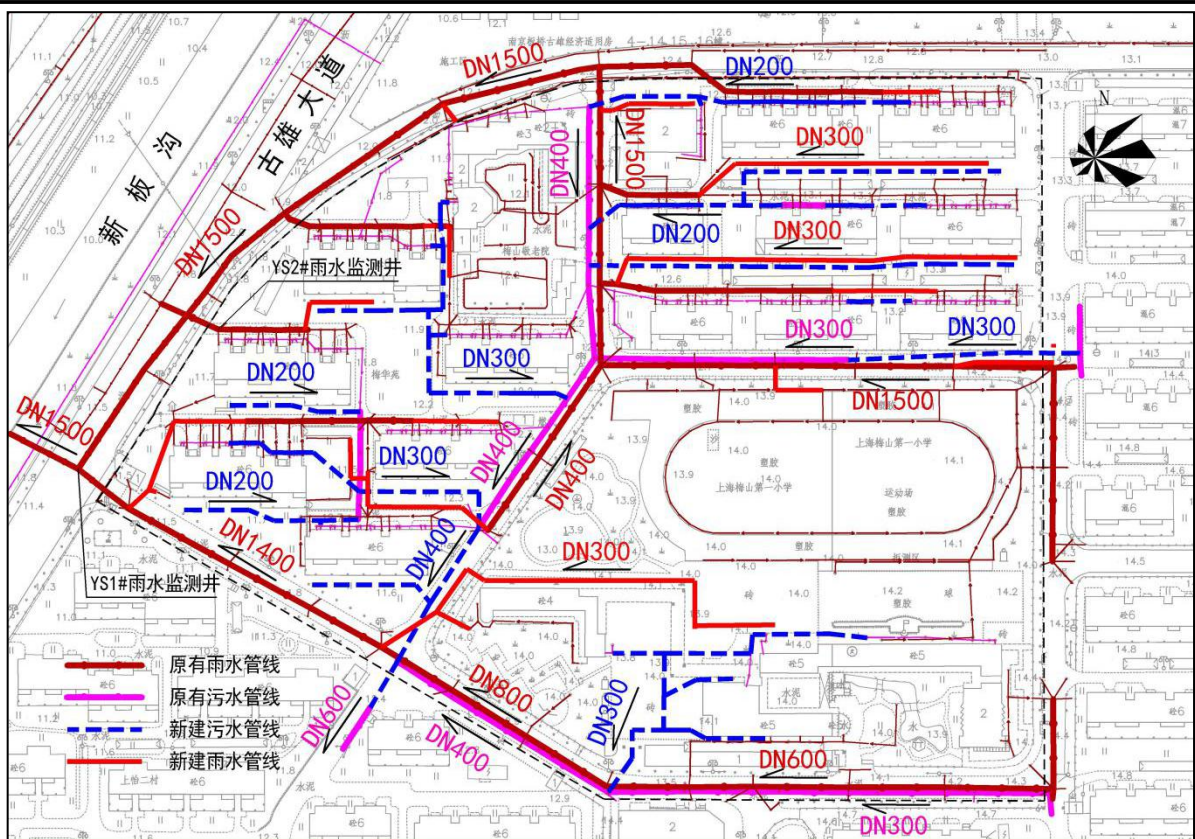
图 2-5 梅华苑排水方案示意图
