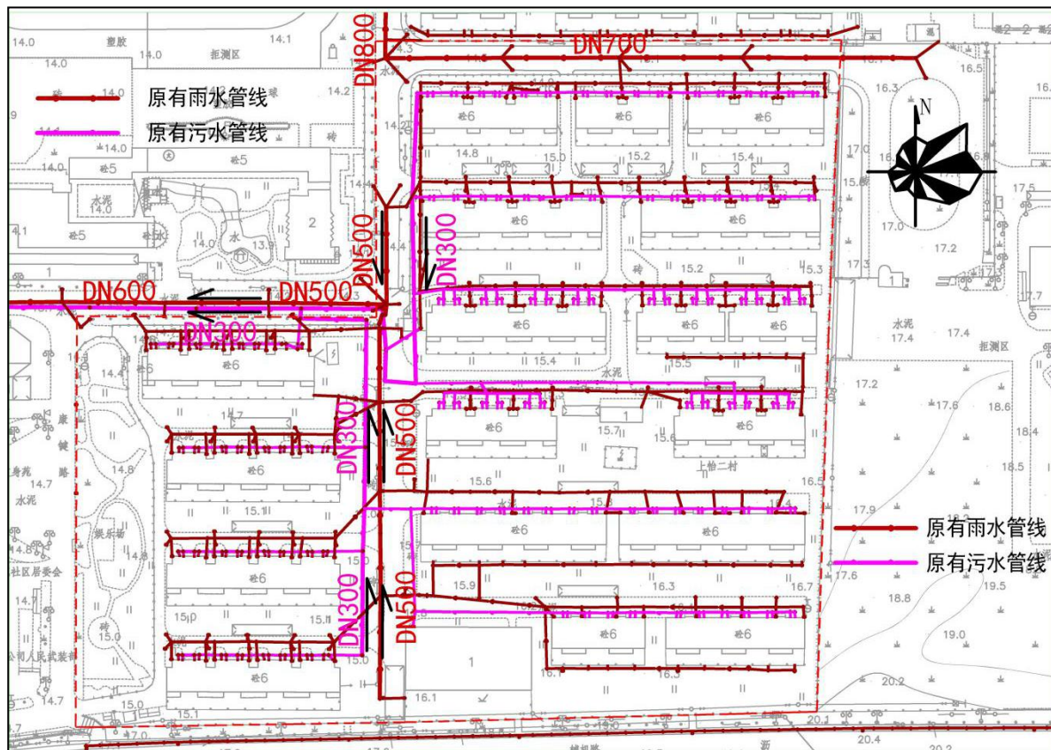
图 2-8 梅盛苑排水现状示意图
