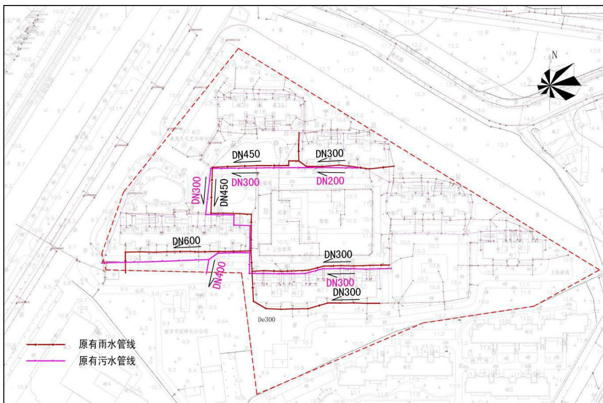
图 2-10 上怡南苑排水现状示意图
