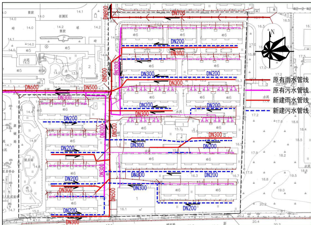
图 2-9 梅盛苑排水方案示意图
