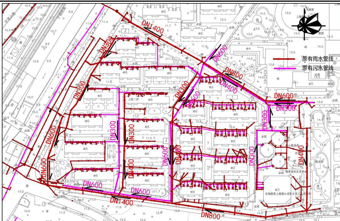
图 2-6 梅秀苑排水现状示意图
