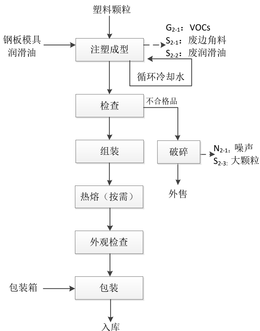
图 5-2 配件制作工艺流程及产污环节图
