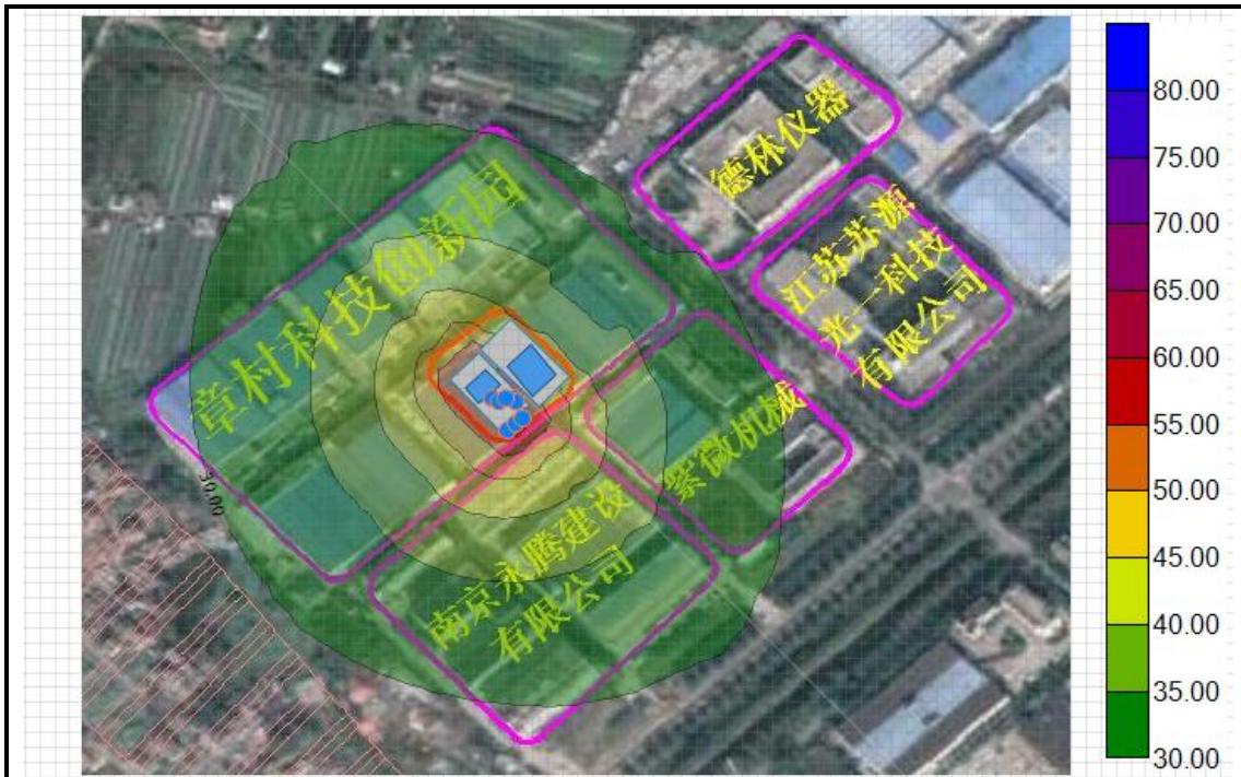
图 7-2 噪声等声级线预测结果图（昼间）
