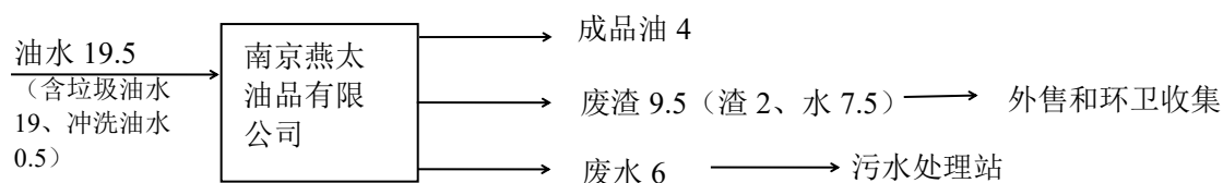
图 4.2-4 本项目油水混合物进南京燕太油品有限公司每天物料平衡图 (t/d)
