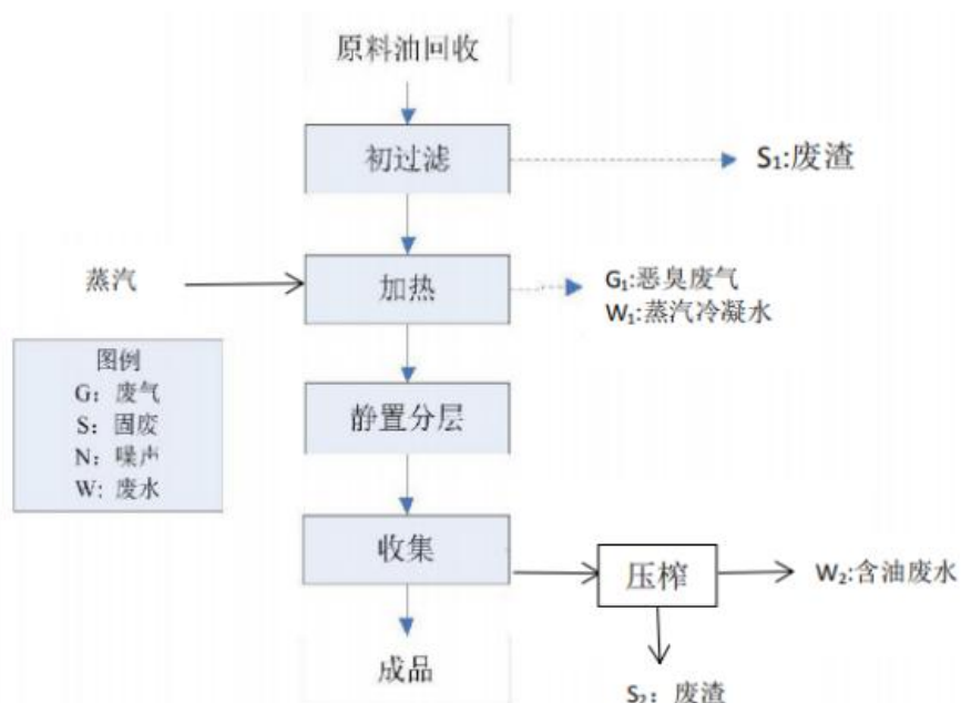
图 3.9-1 南京燕太油品有限公司工艺流程图
