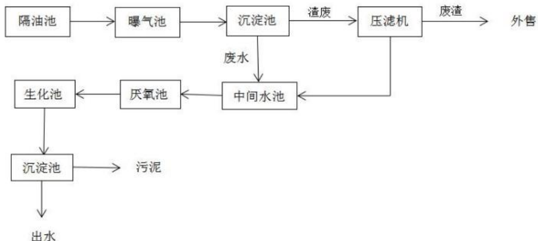
图 3.9-2 南京燕太油品有限公司污水处理工艺
