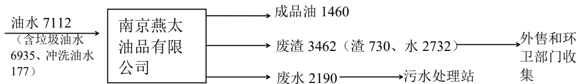
图 7.2-2 油水混合物进南京燕太油品有限公司后物料平衡图（单位：t/a）
