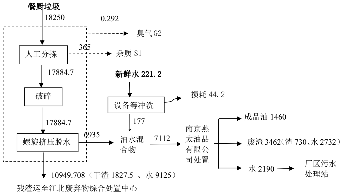
图 4.2-1 本项目餐厨垃圾处置物料平衡图（单位：t/a）
