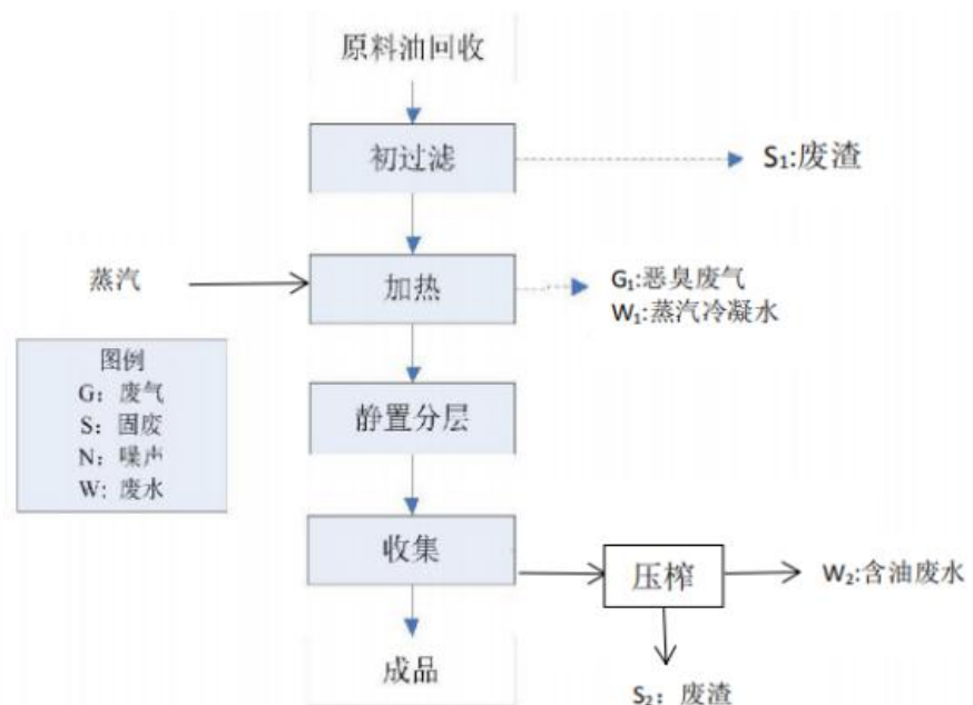
图 7.2-1 油水混合物进南京燕太油品有限公司后的处理流程
