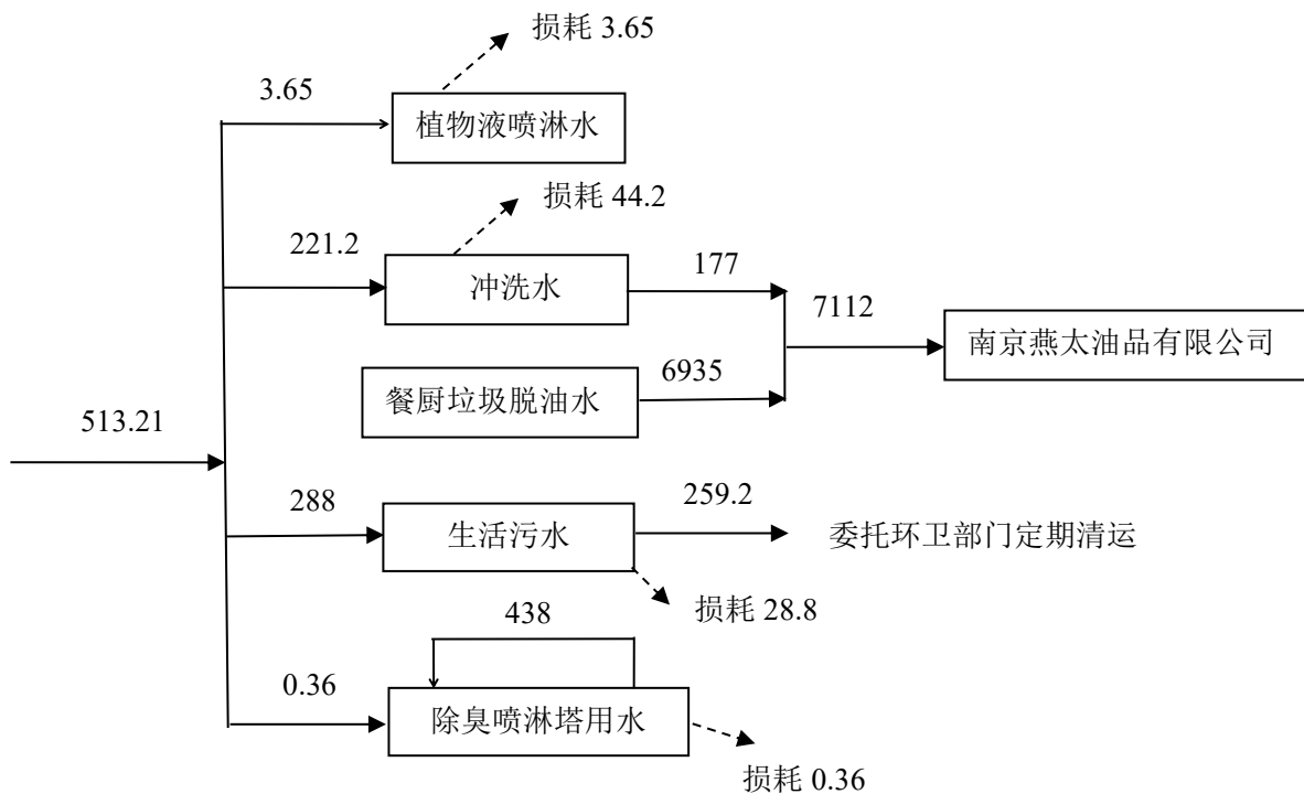
图 4.2-2 建设项目水平衡图（单位：t/a）
