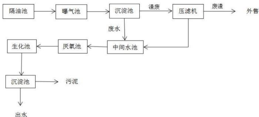
图 7.2-3 南京燕太油品有限公司污水处理工艺
