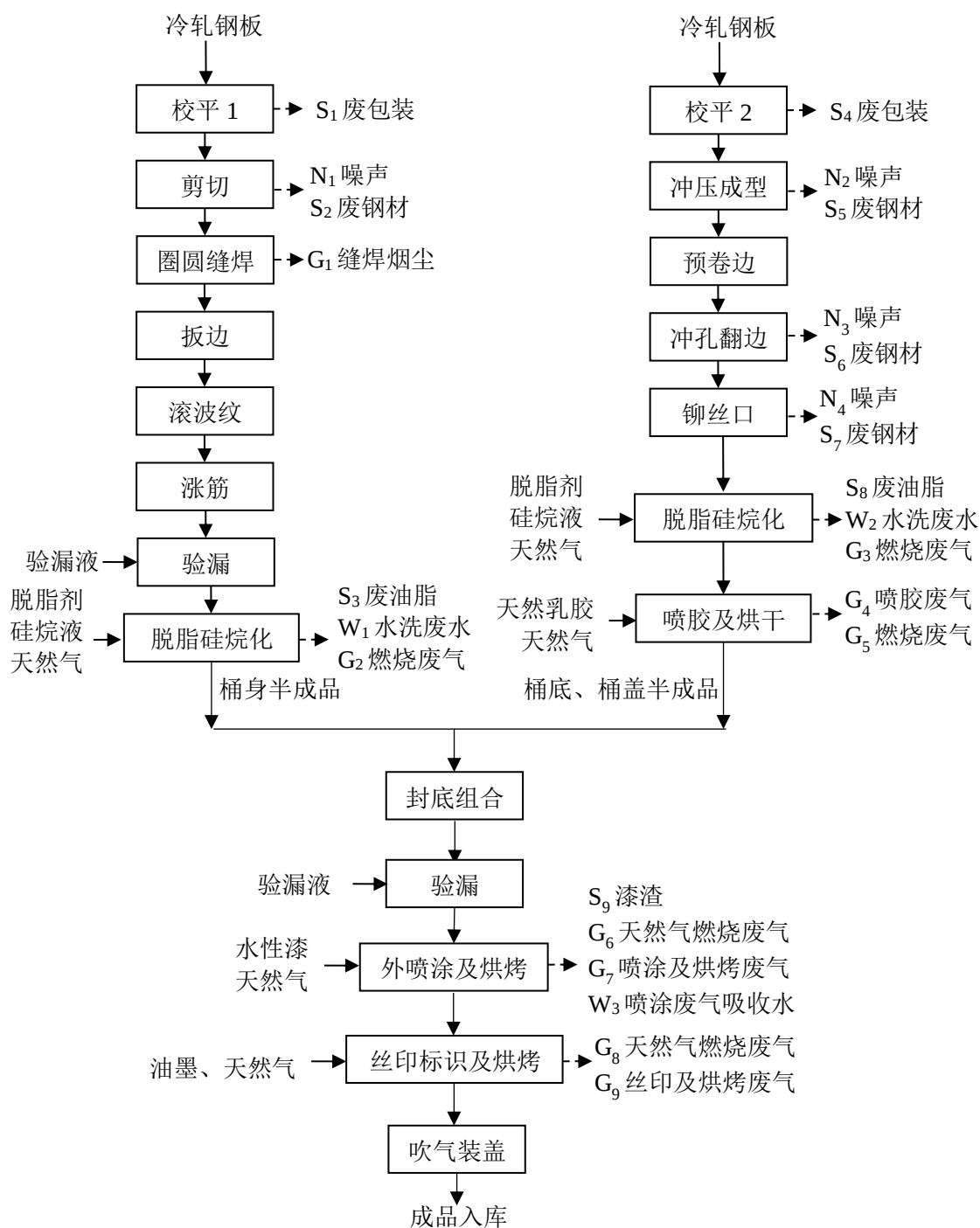
图 2.7-1 全自动钢桶生产线生产工艺流程及产污环节图
