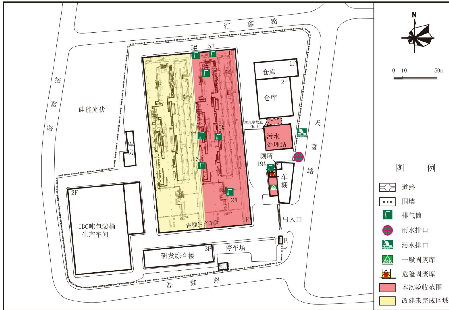
图 2.3-2 平面布置图 (变动后)
